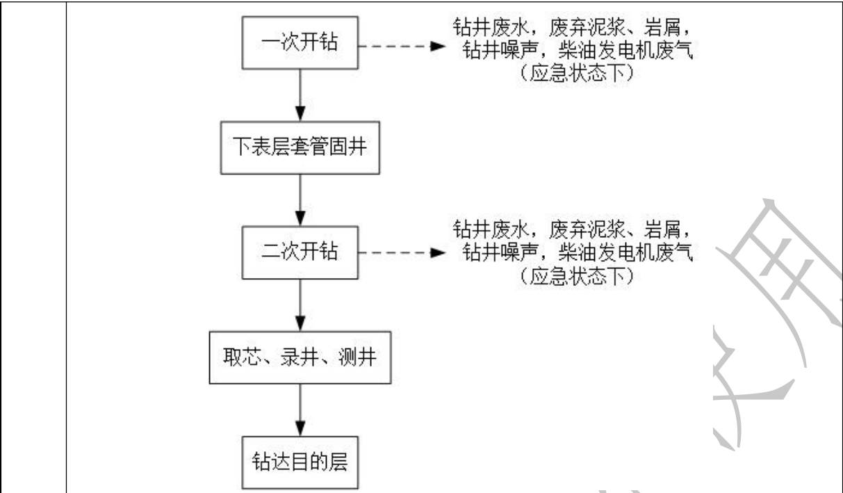
图 2-3 钻井工艺流程图
