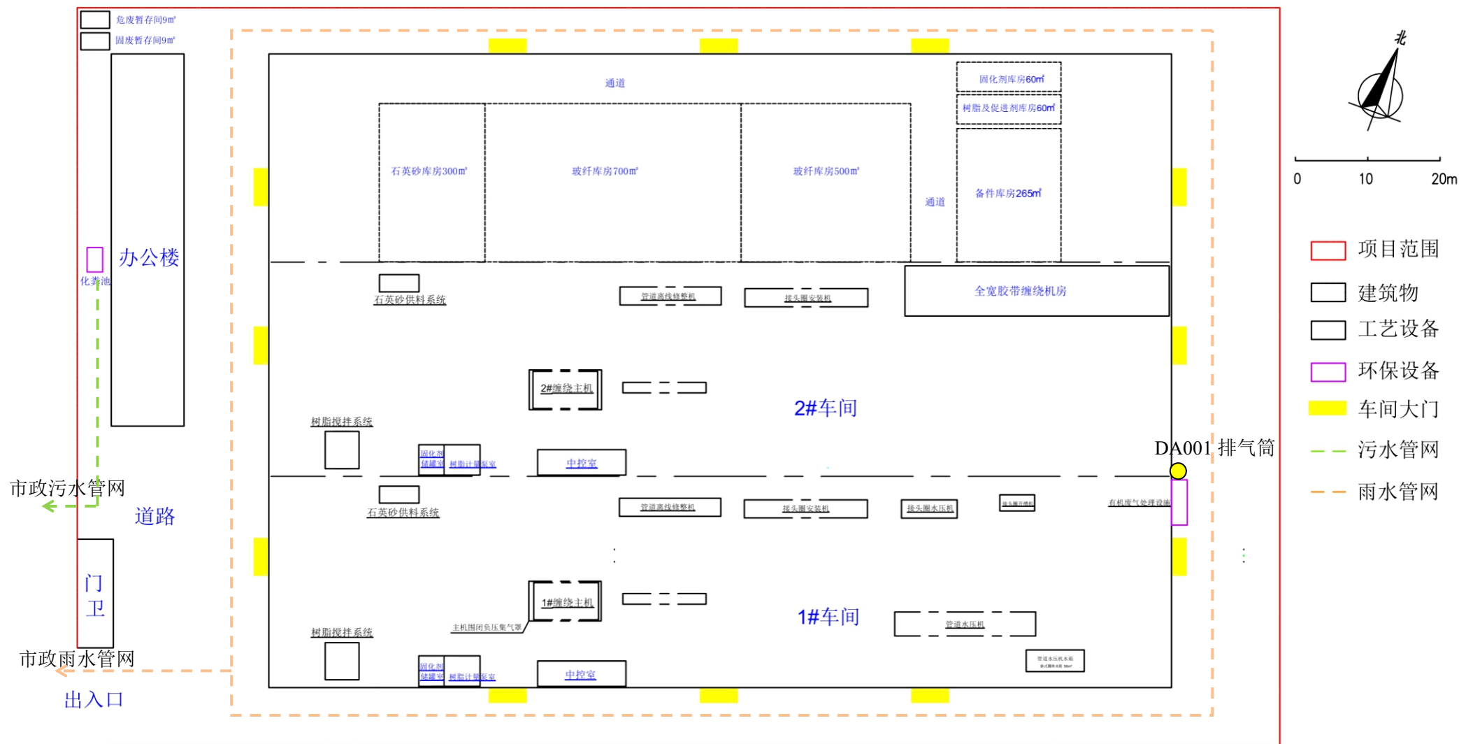
附图 1 平面布置图
