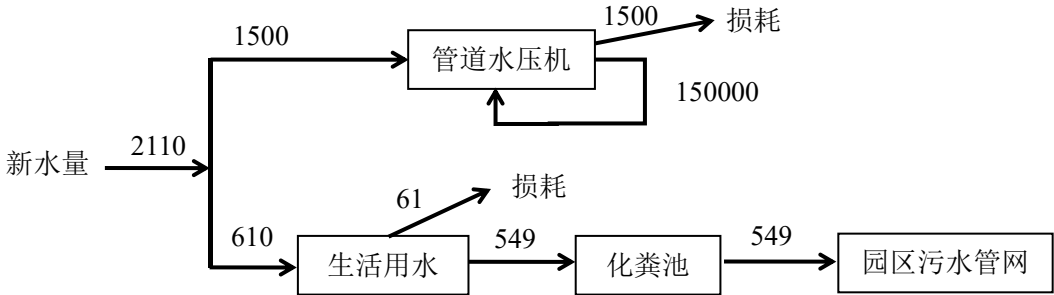
图 2.8-1 水平衡图 (单位 m³/a)
