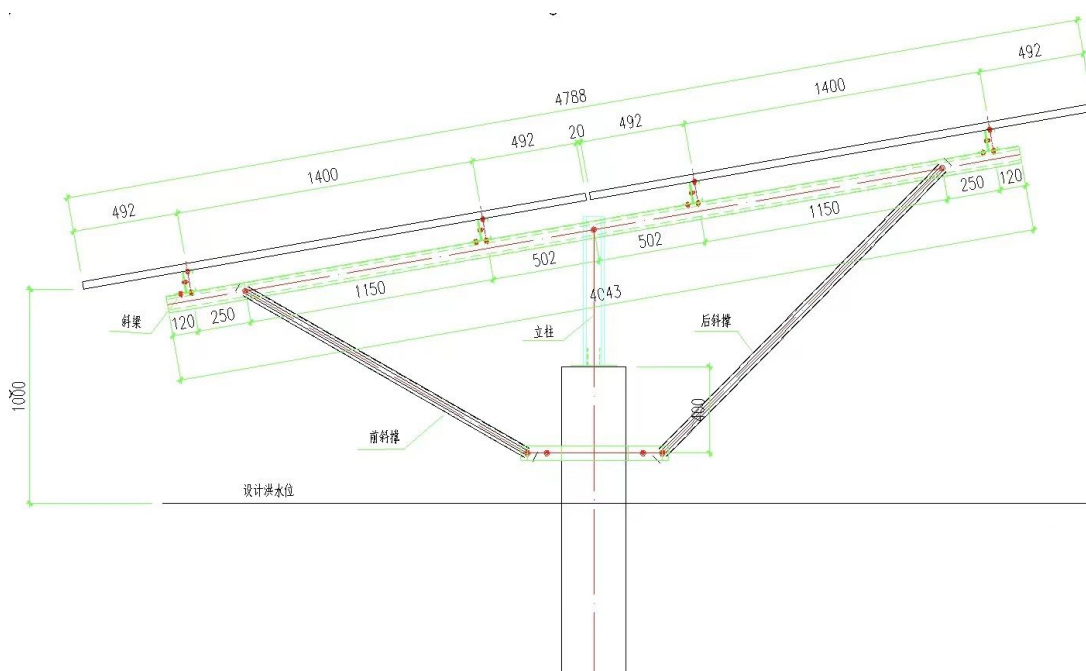
图 2-2 支架剖面图
